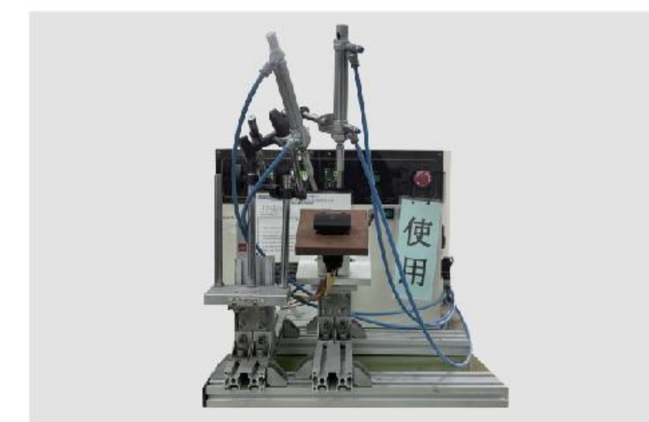
Knob Endurance Tester (For Power Window Switch) 全自動耐久試驗機
